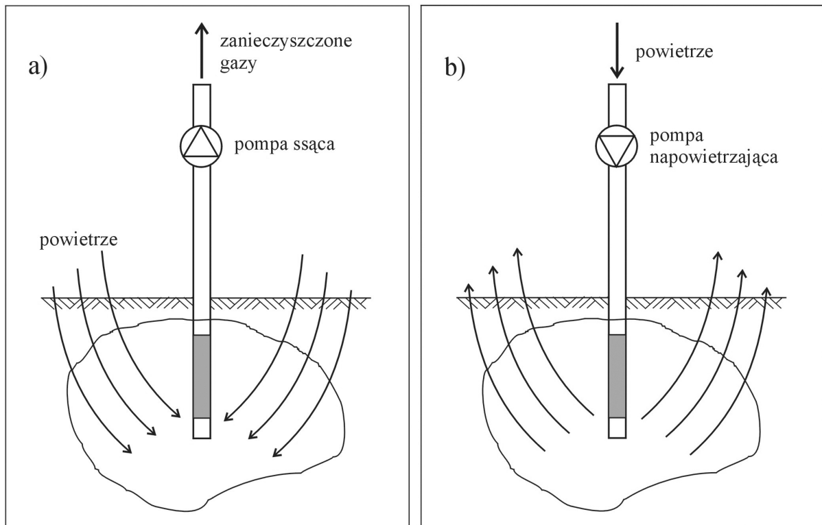
Rys. 1.18. Schemat procesu biowentylacji a) ekstrakcja powietrza gruntowego b) iniekcja powietrza
