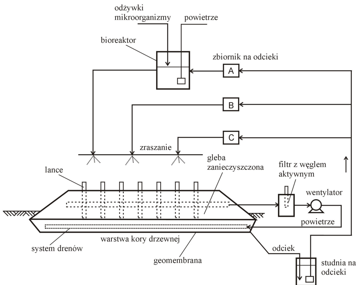
Rys. 1.20. Schemat biologicznego oczyszczania gleby metodą pryzmowania
