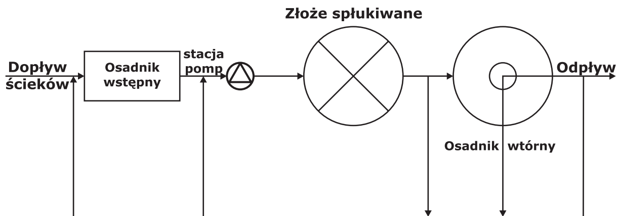
Rys. 2.24. Schemat oczyszczania ścieków na złożach biologicznych
