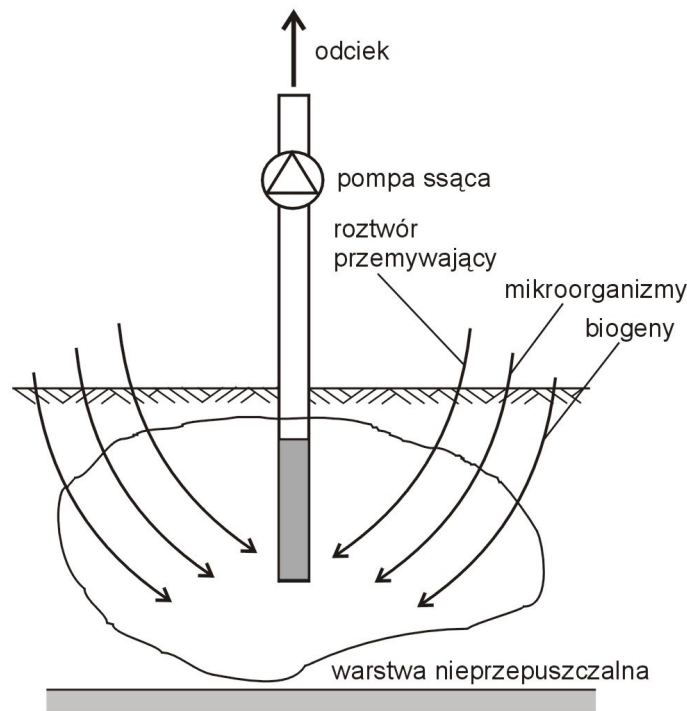
Rys. 1.17. Schemat procesu bioremediacji stymulowanej wodą
