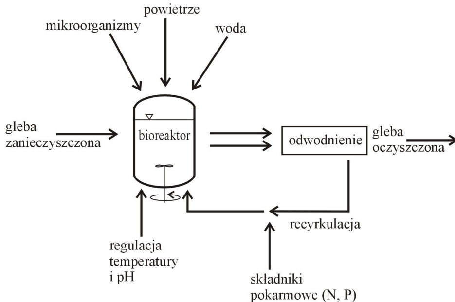
Rys. 1.19. Schemat bioreaktora
