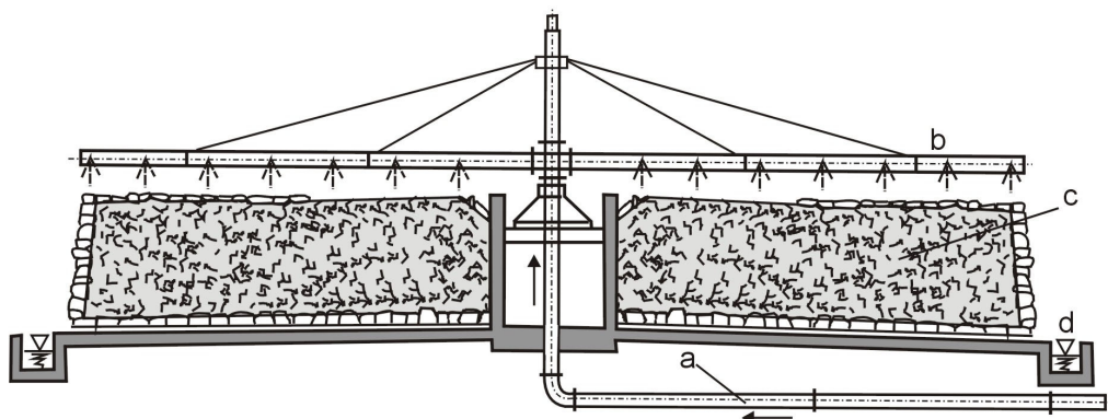
Rys. 2.23. Złoże zraszane: a) dopływ b) urządzenia zraszające c) wypełnienie złoża d) odpływ
