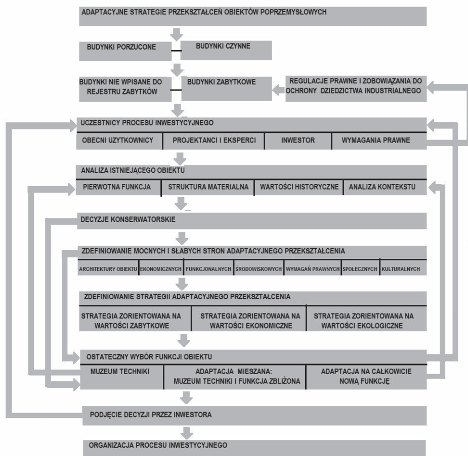
Il. 1. Schemat procesu podejmowania decyzji w przypadku adaptacyjnych przekształceń obiektów poprzemysłowych. (oprac. B. Wórzeczek na podstawie: [2])
