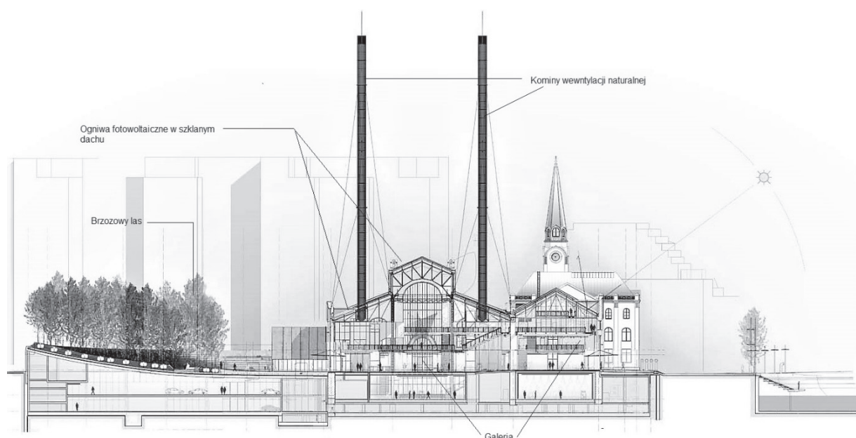
Il. 9. Przekrój przez elektrownię GES2 w Moskwie – elementy ekologiczne w projekcie [25]
