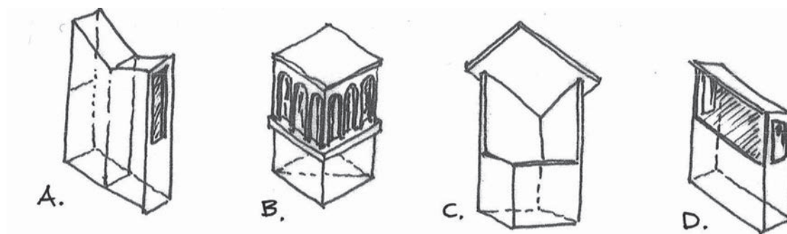
Il. 1. Łapacze wiatru charakterystyczne dla Bliskiego Wschodu i Egiptu (oprac. A. Mielńska na podstawie: [8])
