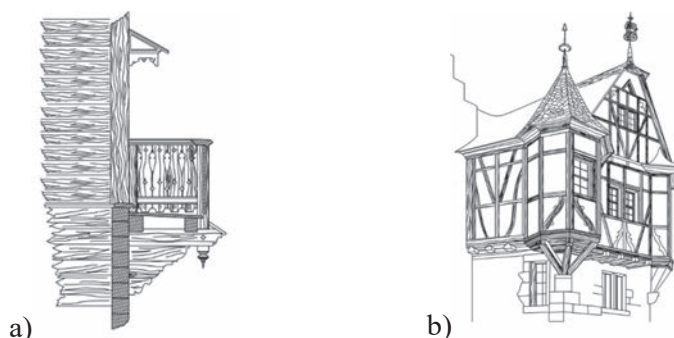
II. 2. Uprozczone schematy konstrukcji wspornika: a) podparcie balkonu wspornikiem z belki wielokrotnej, b) wykusz podparty wspornikami prętowymi, trójkątnymi (oprac. B. Misztal na podstawie: [4 ])
