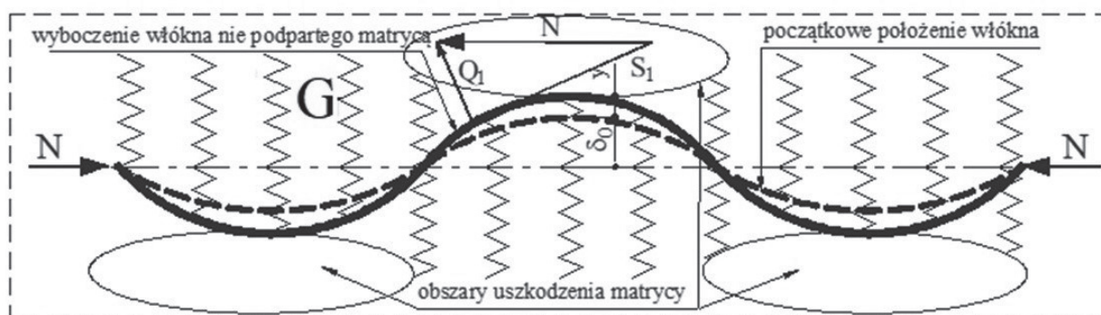
Il. 4. Wyboczenie włókna ściskanego obarczonego wstępnym wygięciem \delta_0 w ośrodku lepkosprężystym (oprac. B. Misztal)
