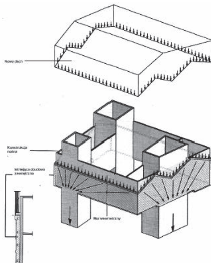
Il. 7. Struktura konstrukcyjno-budowlana nowej i historycznej obudowy CaixaForum w Madrycie (oprac. B. Wórzeczka na podstawie: [20])
