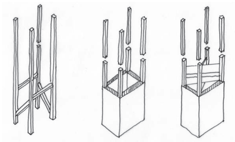
Il. 8. Prętowa konstrukcja drewniana, wzmacniająca ściany murowane łapacza wiatru. (oprac. A. Mielńska na podstawie: [10])
